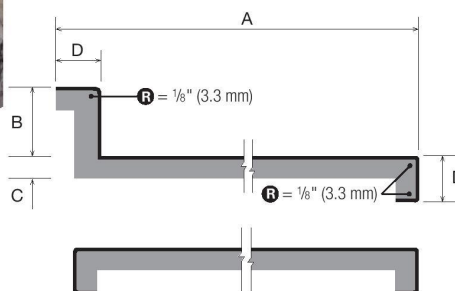
COMPTOIR AVEC DOSSERET / COUNTERTOP WITH BACKSPLASH DIMENSION
